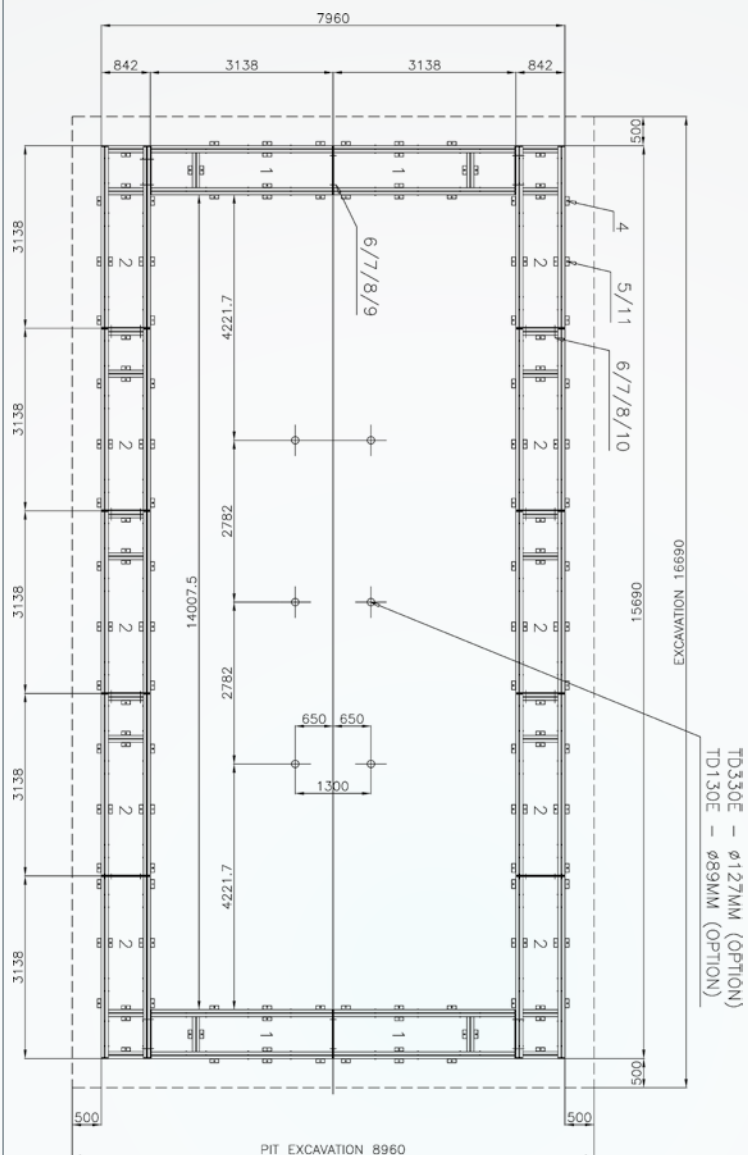
KOREK® FRAME - CHASSIS KOREK® KOREK® RAHMEN - KOREK® PAMA - 16 M X 8 M
