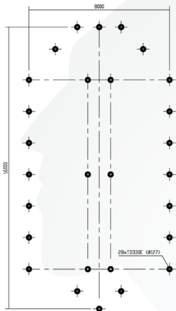
16 M X 8 M TD 330E / TD130E
